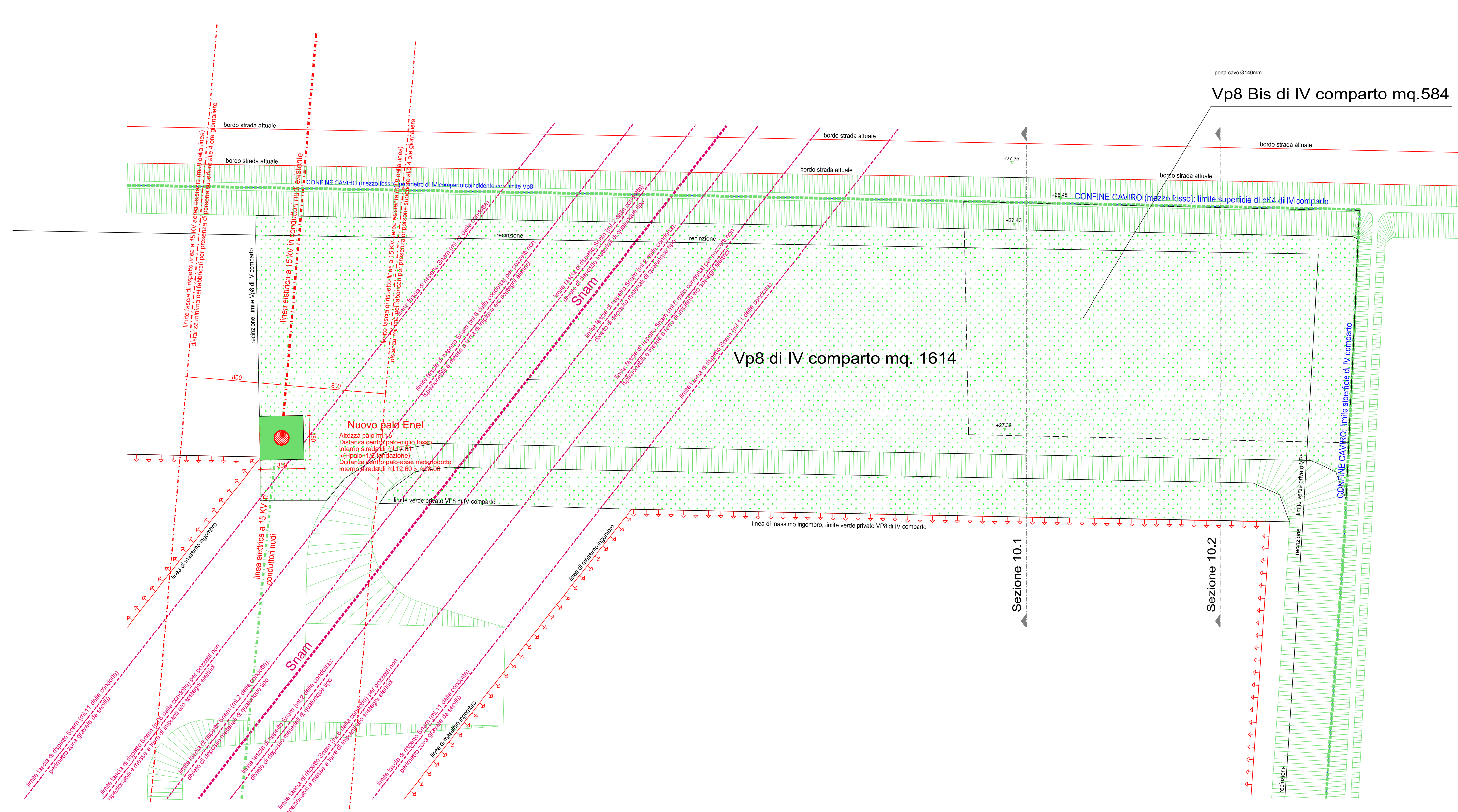
Stato modificato scala 1:200
