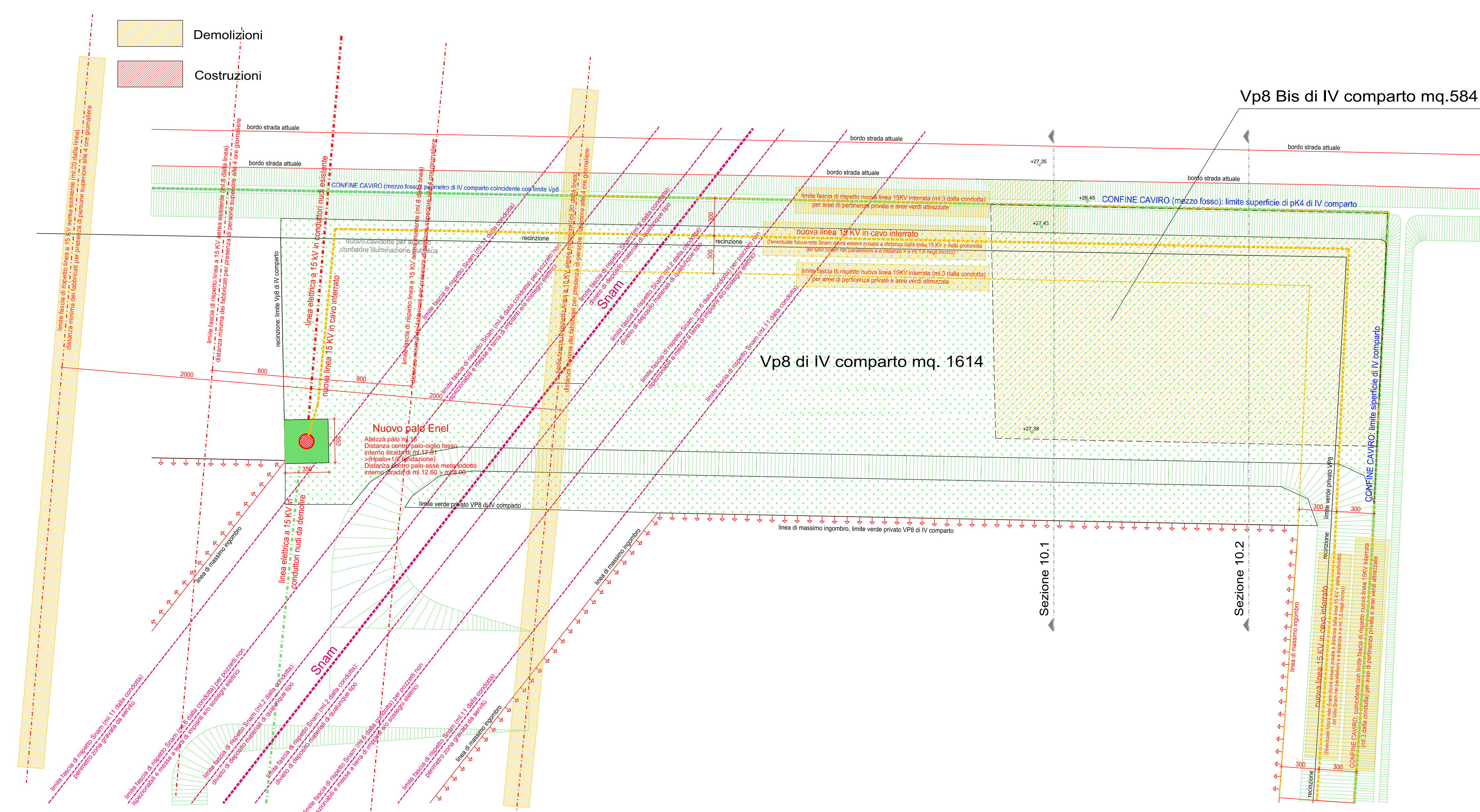
Stato comparato scala 1:200
